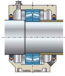
Filzstreifendichtung SC..FS
