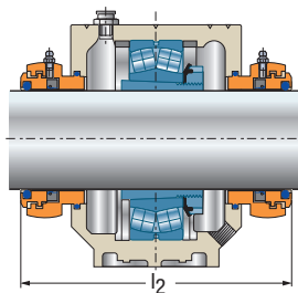
Taconite-Dichtung SC..TA
