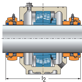
Taconite-Dichtung SC..TA
