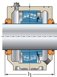
Labyrinthdichtung SC..LA
