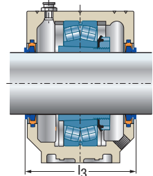
Filzstreifendichtung SC..FS + V-Ring V..A
